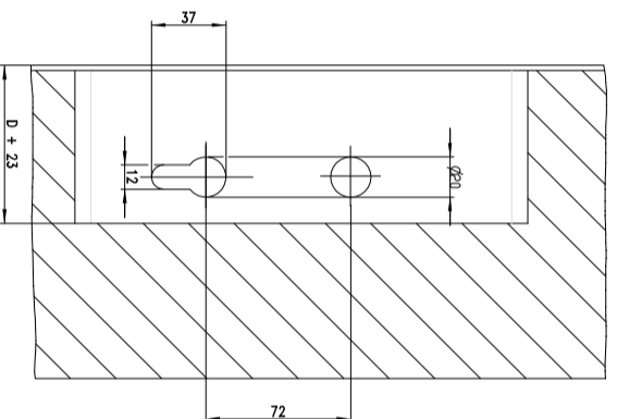
Frezing voor de Hoofdslootkast
