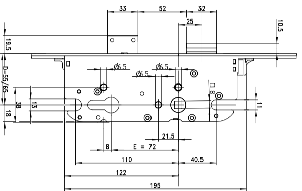
Maatvoering hoofdslootkast
