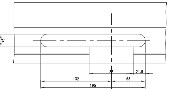
Frezing in kozijn voor sluitkorn hoofdsloot
