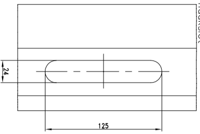
Frezing in het kozijn voor sluitkorn haaksloot
