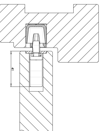
Sluithaak
