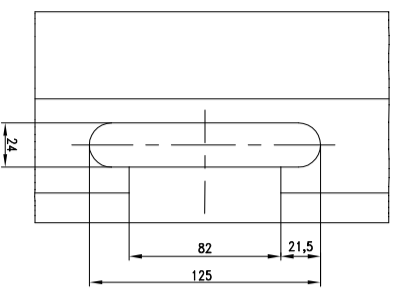
Frezing in het kozijn voor sluitkom automatische schoot
