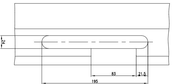
Frezing in kozijn voor sluitkom hoofdslot
