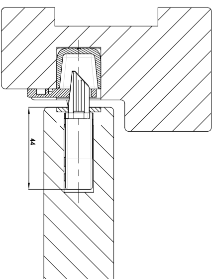
Automatische schoot
