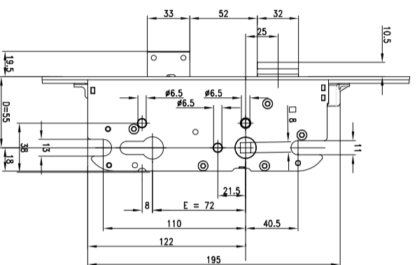
Maatvoering hoofdslotkast
