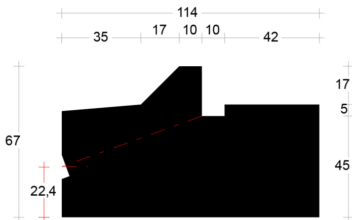
Onderdorpel BI sponning 52mm (art. 2045389)
