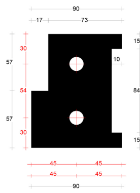
Eindneut rechts 90mm art. 2045617
