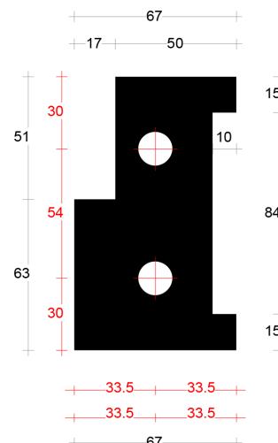
Neut rechts 67mm art. 2045411
