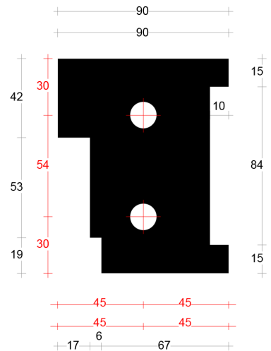
Neut rechts 90mm art. 2045470
