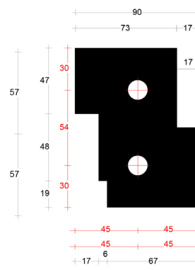
Tussenneut rechts 90mm art. 2045615
