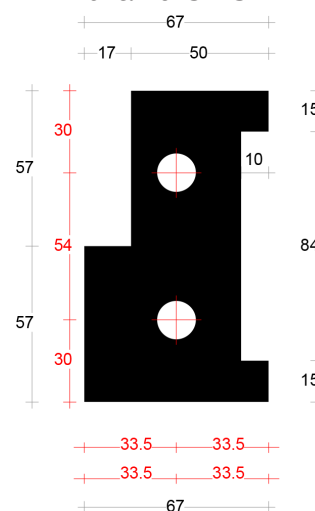
Neut rechts 67mm 1 art. 2045413
