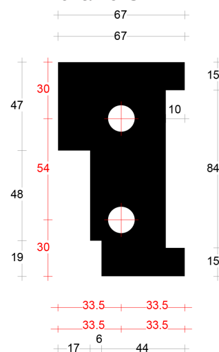
Neut rechts 67mm 1 art. 2045421
