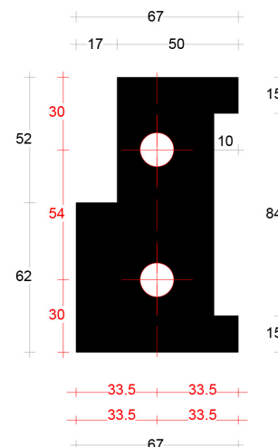
Neut rechts 67mm art. 2045376
