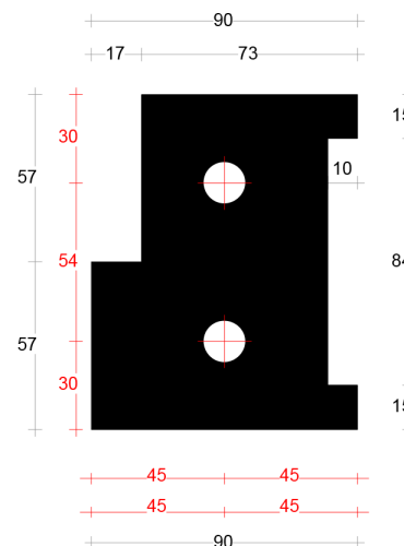
Neut rechts 90mm art. 2045438
