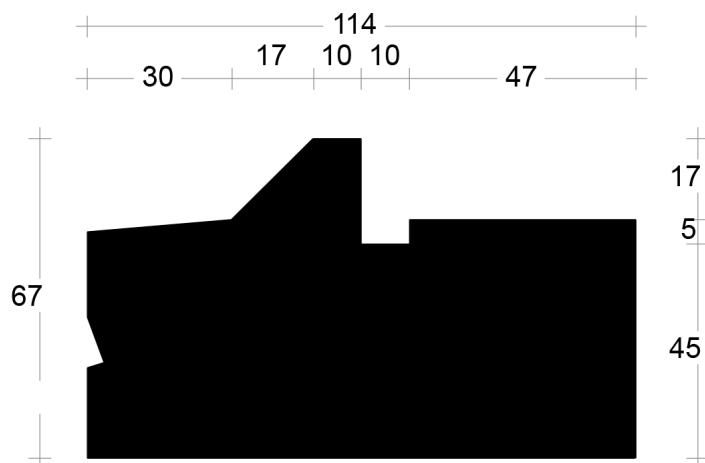
Onderdorpel BI sponning 57mm (art. 2045401)
