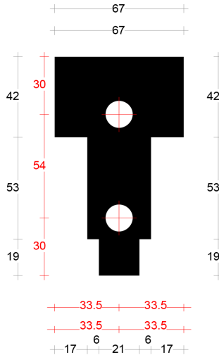
Tussenstijlneut 67mm art. 2045468
