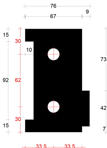
Neut vaste deur links art. 2045456
