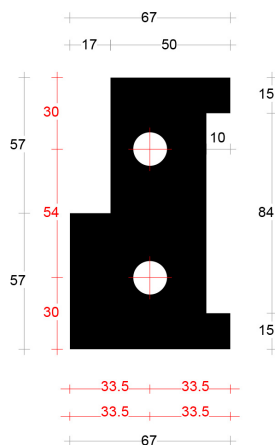
Eindneut rechts 67mm art. 2045613
