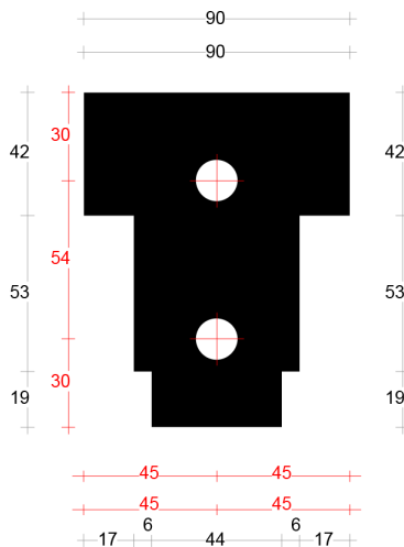
Tussenstijlneut 90mm art. 2045471
