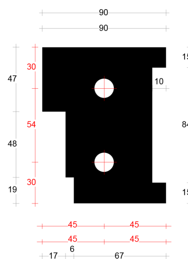
Neut rechts 90mm art. 2045386
