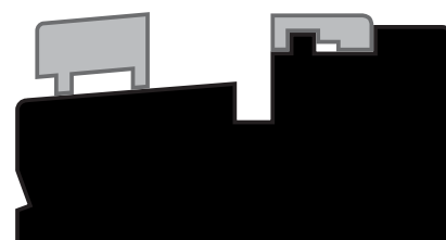
BU-glaslat 20x30mm (art. 2045451 ) op BU-onderdorpel
