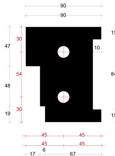
Neut rechts 90mm art. 2045431
