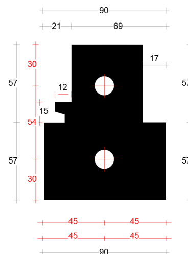
Tussenstijlneut rechts 90mm art. 2045394
