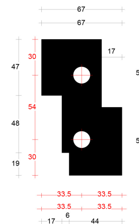
Tussenneut rechts 67mm art. 2045611
