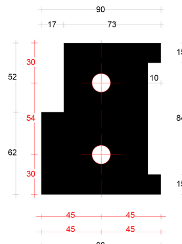
Neut rechts 90mm art. 2045379
