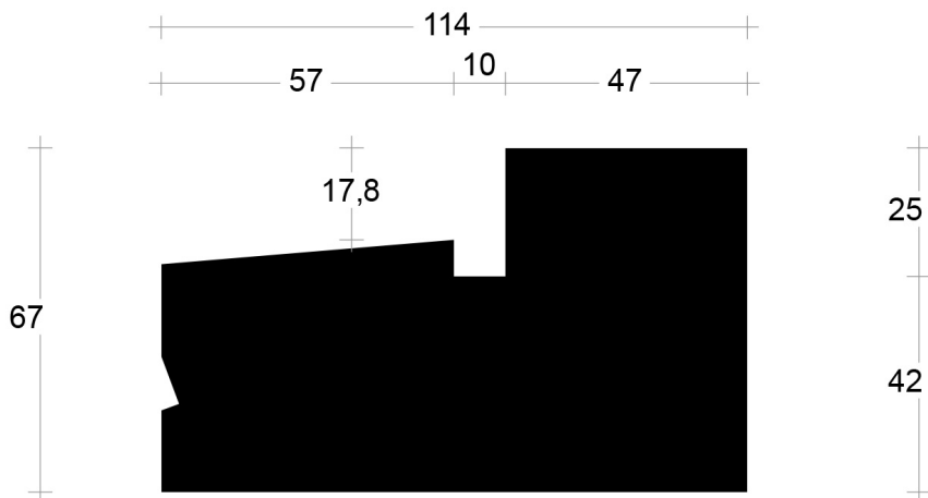
Onderdorpel BU VD 17 sponning 67mm (art. 2045381)
