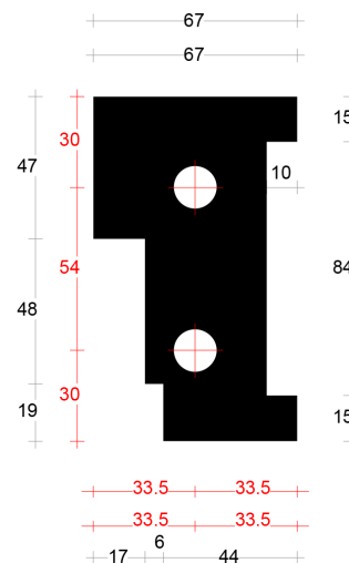
Neut rechts 67mm art. 2045421
