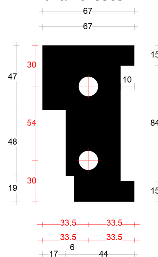
Neut rechts 67mm art. 2045383
