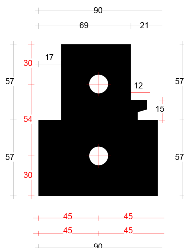
Tussenstijlneut links 90mm art. 2045393
