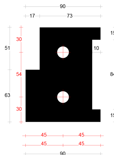
Neut rechts 90mm art. 2045433
