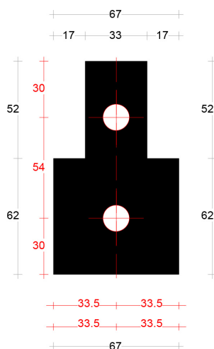
Tussenstijlneut 67mm art. 2045377
