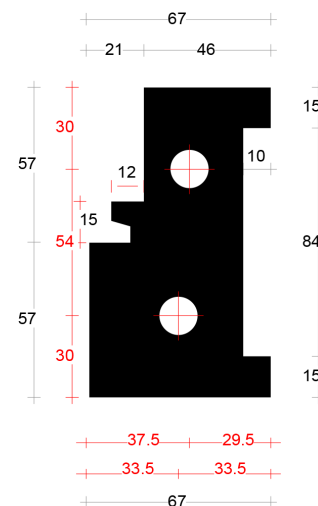
Neut rechts 67mm art. 2045391
