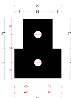
Tussenneut 90mm art. 2045618
