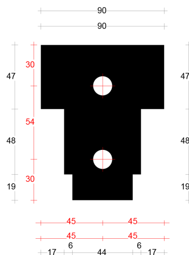
Tussenstijlneut 90mm art. 2045435
